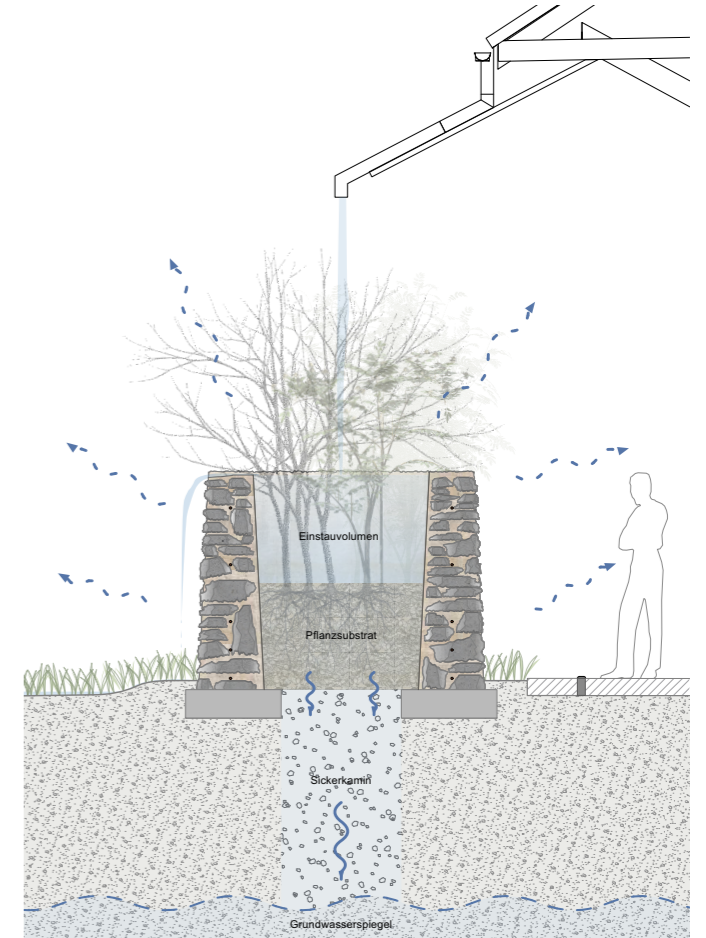
Schnitt Sickertopf
