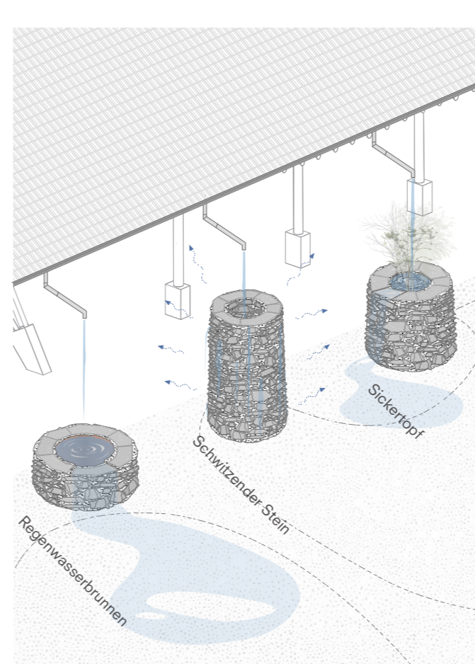
Typologie Sickertopf
